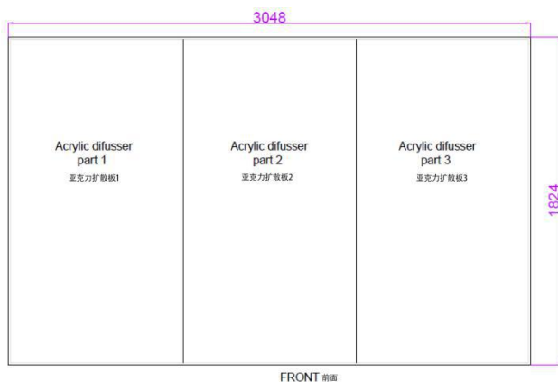
FRONT 前面
