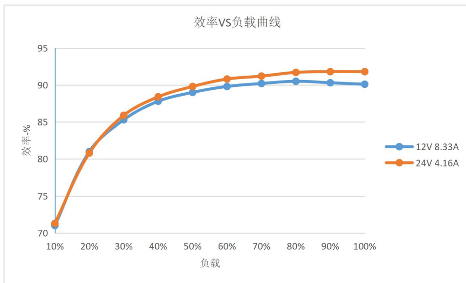
效率VS负载
