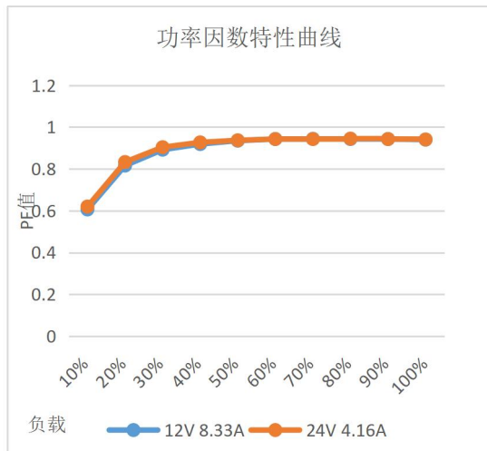
功率因数特性曲线
