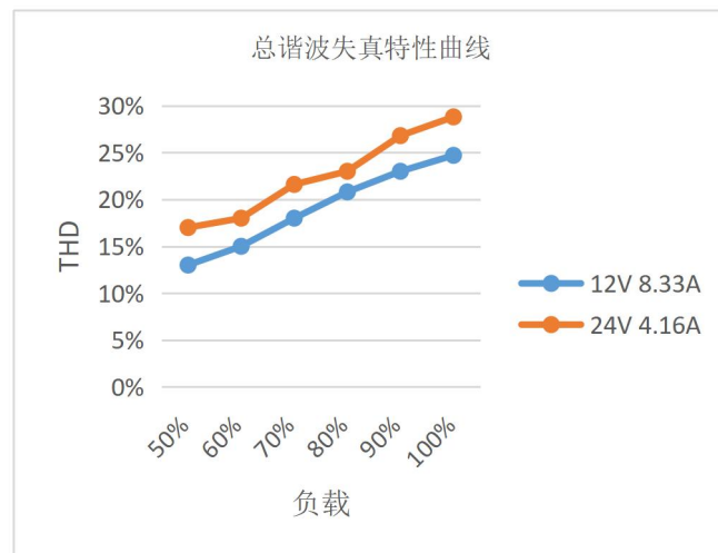
总谐波失真特性曲线
