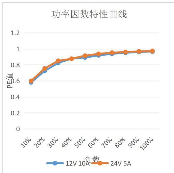
功率因数特性曲线
