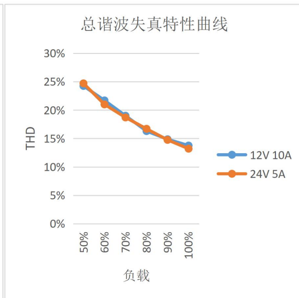
总谐波失真特性曲线
