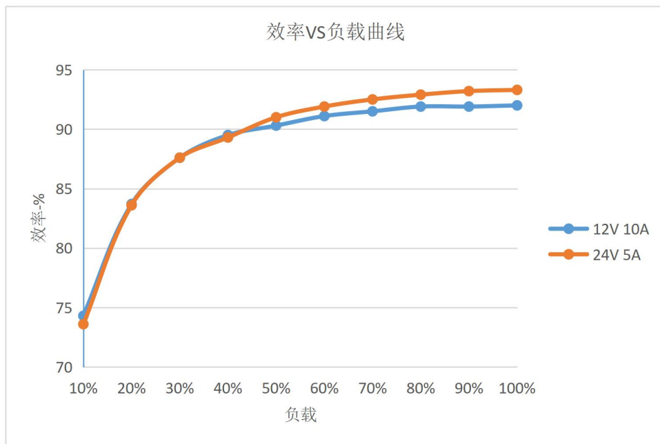
效率VS负载
